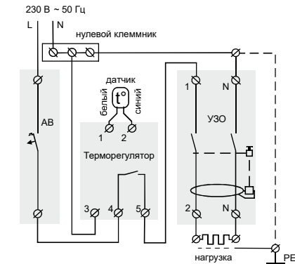
Схема 1. Подключение АВ и УЗО
